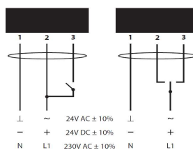
Электрическое подключение
