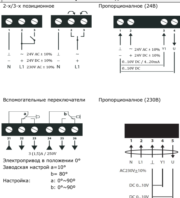
Электрическое подключение
