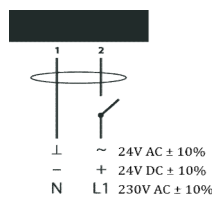
Электрическое подключение
