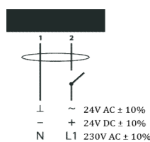
Электрическое подключение
