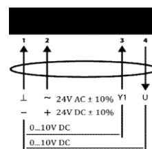
Электрическое подключение
